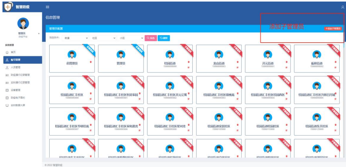
账号管理 1
